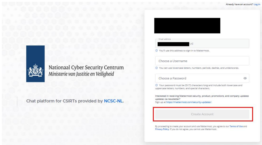
Figuur 2: Loginscherm
