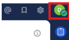
Figuur 5: Gebruikersinstellingen
