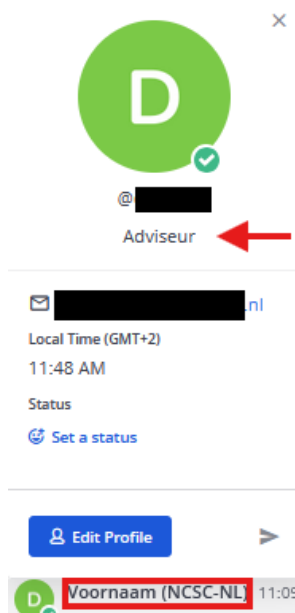
Figuur 10: Functiebeschrijving
