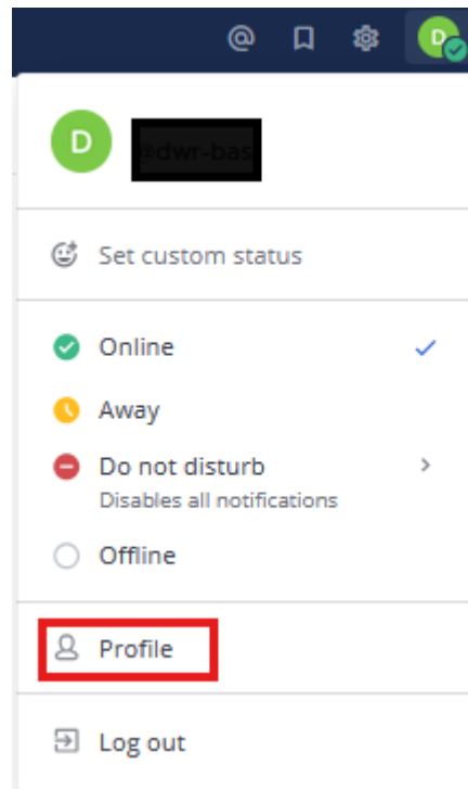
Figuur 6: Gebruikersprofiel
